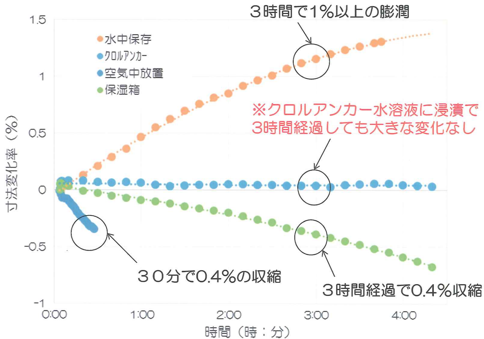
アルギン酸塩印象材の寸法変化
