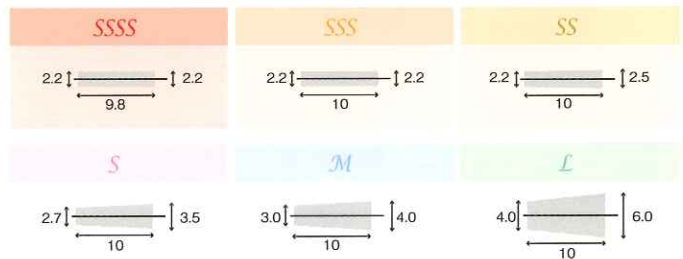
●ブラシ部分サイズ (単位 mm)
